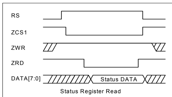
图 6-7：状态读取
