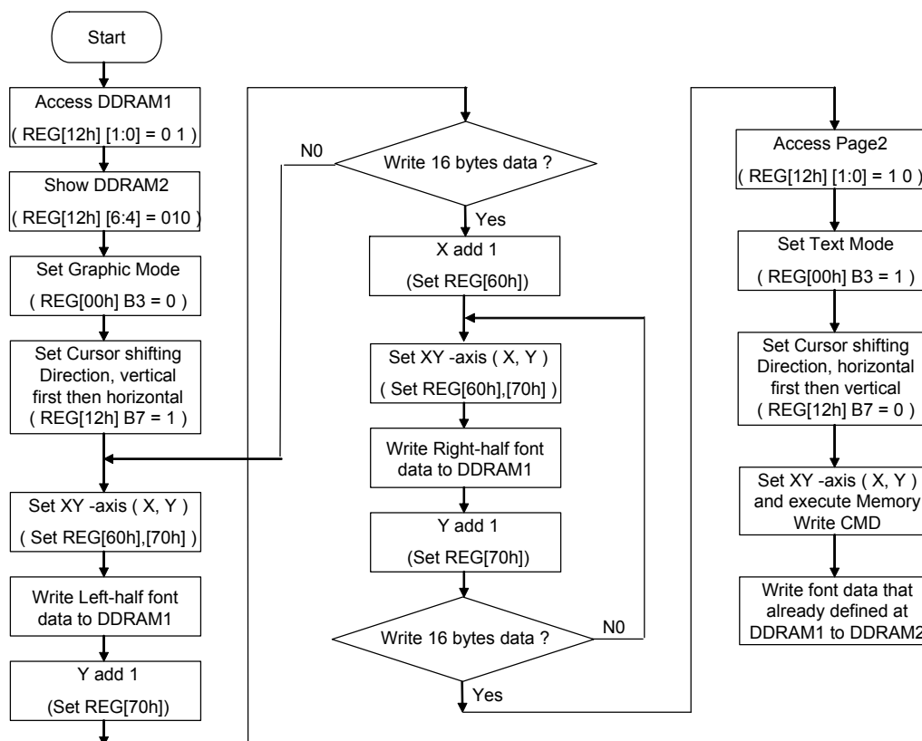
图 6-54 : 在 DDRAM1 创造字型的流程图
