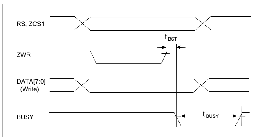
图 6-36 : BUSY 时序图
