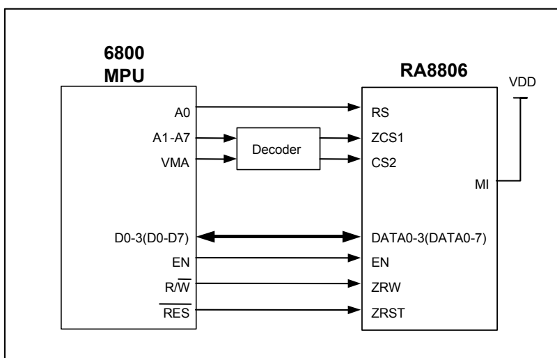
图 6-2 : 6800 (4/8-位) MPU 接口
