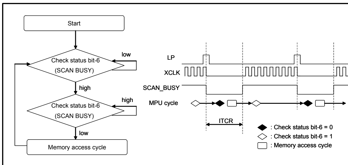
图 6-76 : 以 Check BUSY 来消除雪花 ideal 状况 (2)
