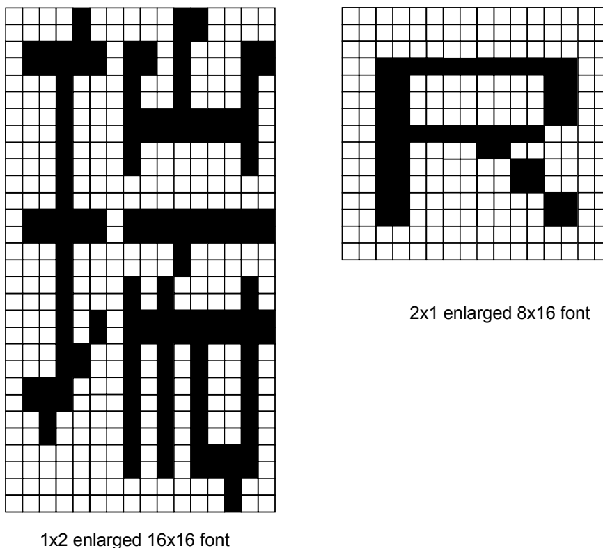
图 6-49 : Font Size Adjustment
