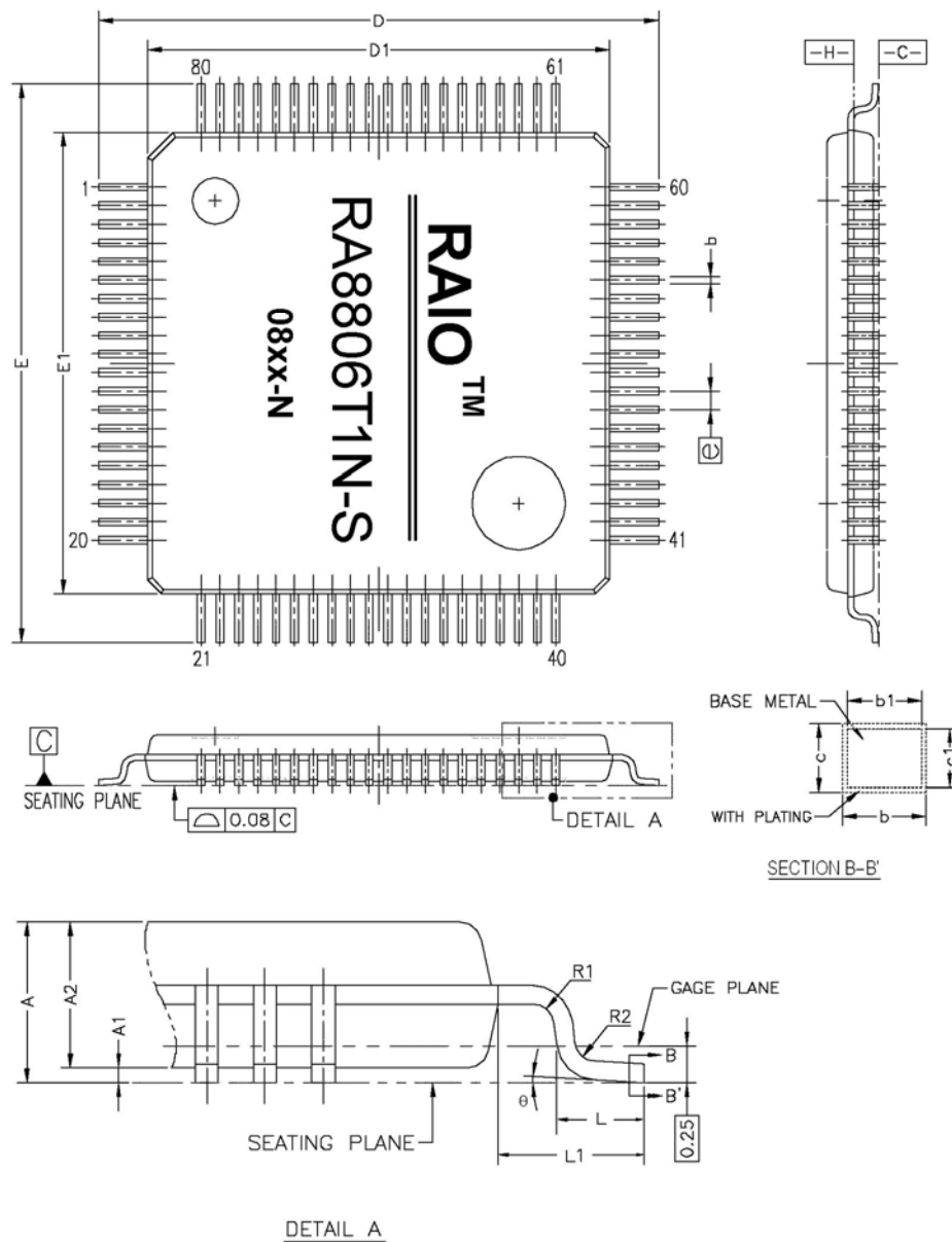
图 7-5 : TQFP-80Pin 机构图
